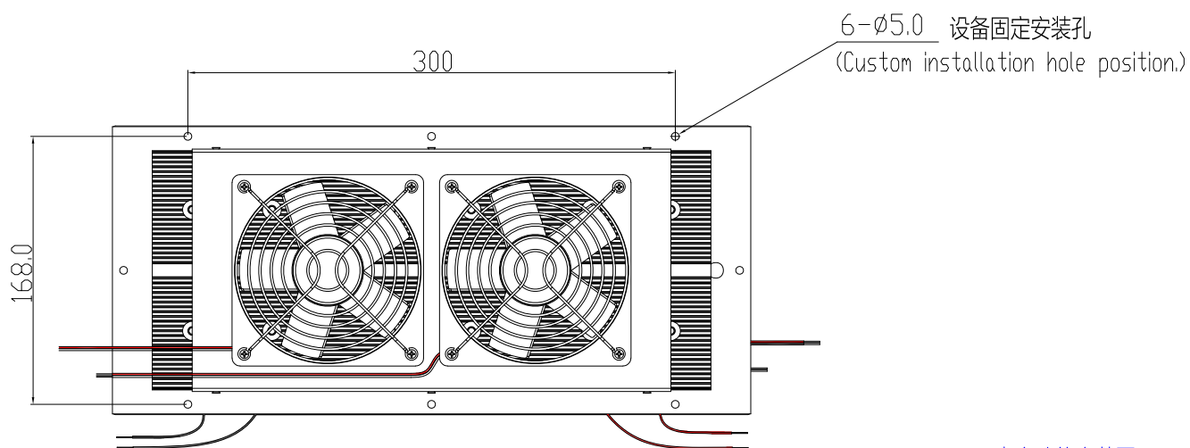
客户孔位安装图
