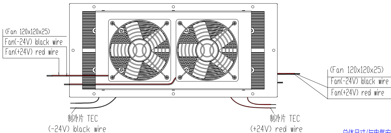
总体尺寸/与电气安装图
