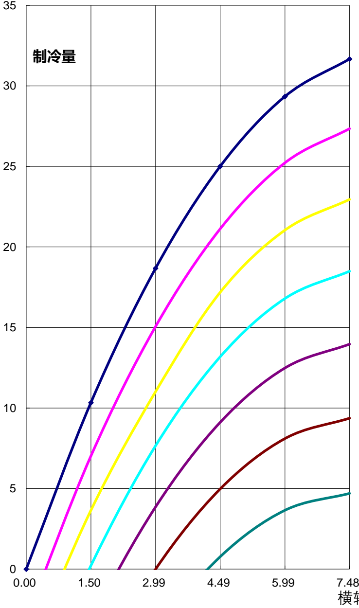
制冷量/电流曲线
